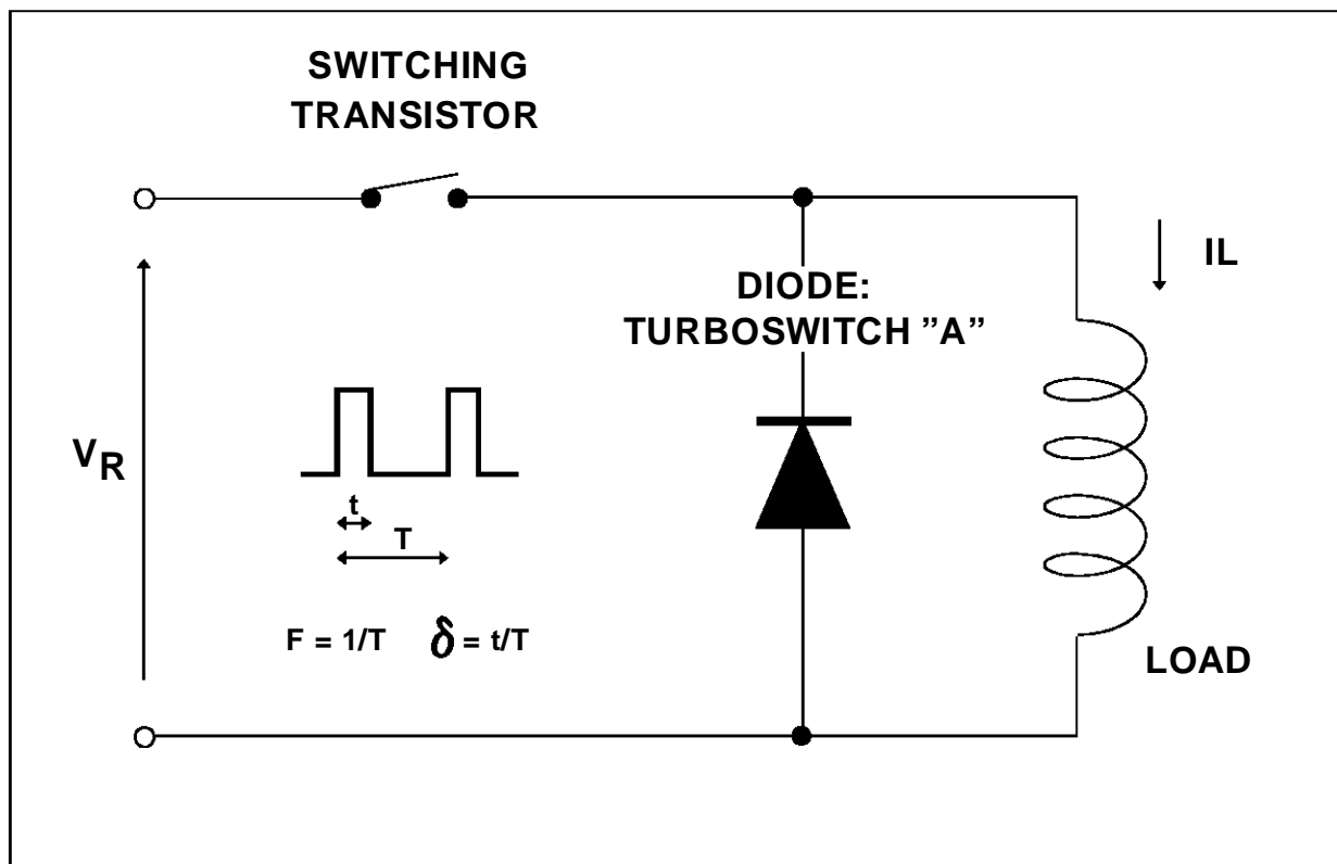
Fig. 1 : "FREEWHEEL MODE".
